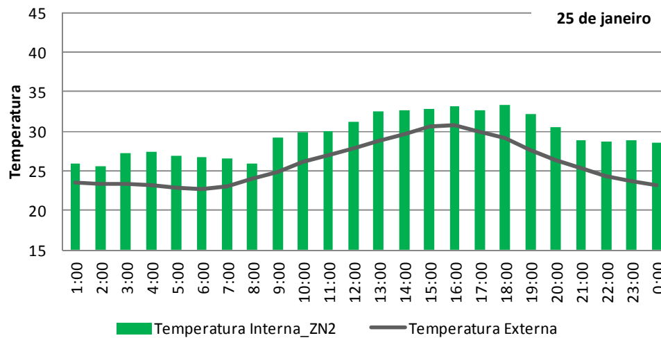
Figura 23 - Temperatura interna da Zona 2 com o uso da ventilação natural.
