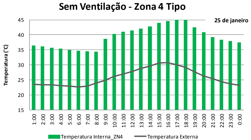
Figura 28 - Temperatura interna da Zona 4 sem o uso da ventilação natural.
