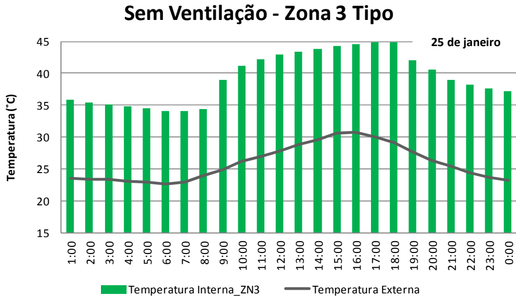
Figura 26 - Temperatura interna da Zona 3 sem o uso da ventilação natural.
