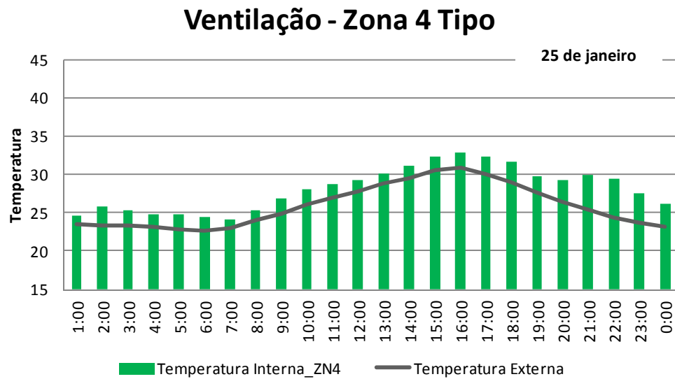
Figura 27 - Temperatura interna da Zona 4 com o uso da ventilação natural.
