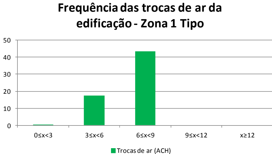
Figura 30 - Frequência de ocorrência das trocas de ar – Zona 1.
