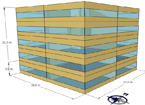
Figura 20 – Modelo comercial com 5 pavimentos.
