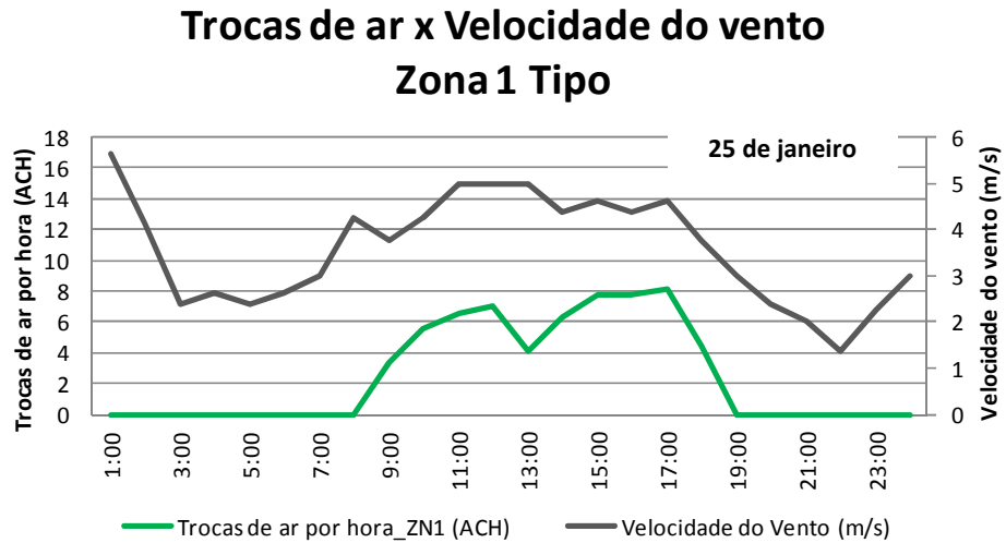
Figura 29 - Análise da velocidade do vento e trocas de ar da Zona 1.
