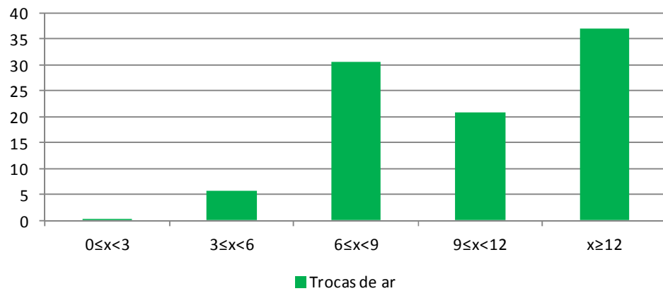
Figura 32 - Análise da velocidade do vento e trocas de ar da Zona 2.
