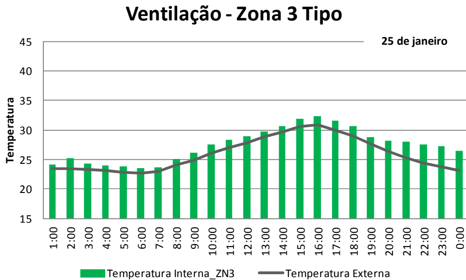
Figura 25 - Temperatura interna da Zona 3 com o uso da ventilação natural.
