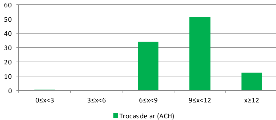
Figura 36 - Análise da velocidade do vento e trocas de ar da Zona 4.
