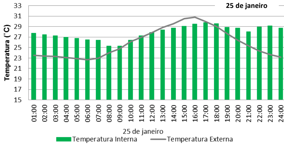
Figura 12 – Temperatura interna da Sala com o uso da ventilação natural.
