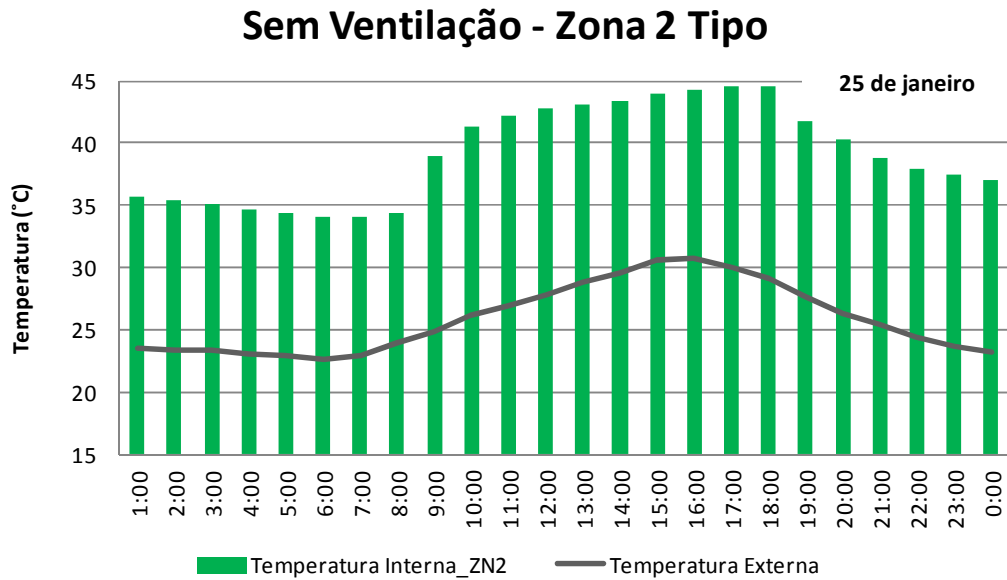
Figura 24 - Temperatura interna da Zona 2 sem o uso da ventilação natural.
