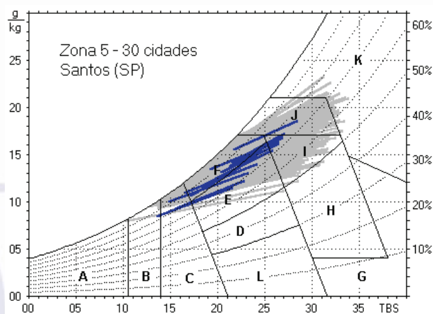
Figura 11 — Carta bioclimática apresentando as normas climatológicas de cidades desta zona, destacando a cidade de Santos, SP
