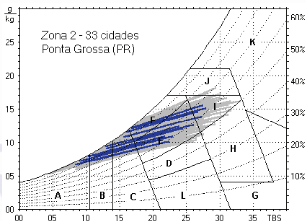
Figura 5 — Carta bioclimática apresentando as normas climatológicas de cidades desta zona, destacando a cidade de Ponta Grossa, PR
