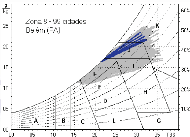
Figura 17 — Carta bioclimática apresentando as normais climatológicas de cidades desta zona, destacando a cidade de Belém, PA
