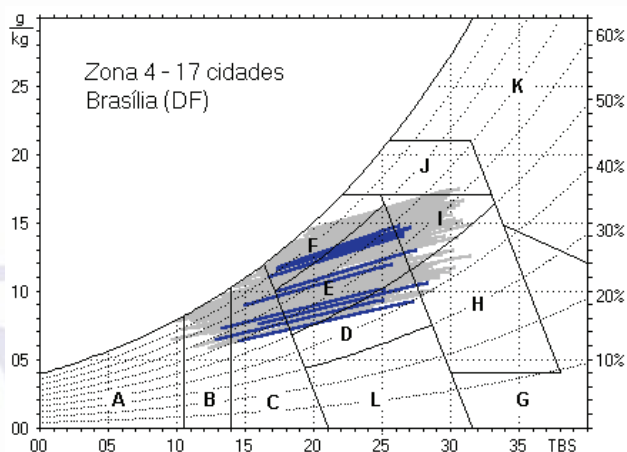
Figura 9 — Carta bioclimática apresentando as normas climatológicas de cidades desta zona, destacando a cidade de Brasília, DF
