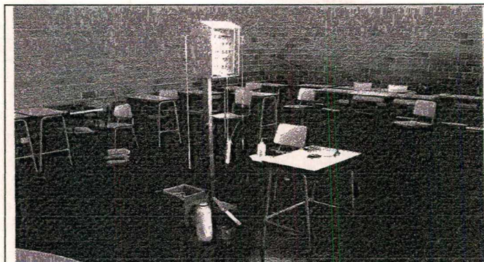
Figura 3.9- Conjunto para a Medição Hígro-Térmica e do vento
