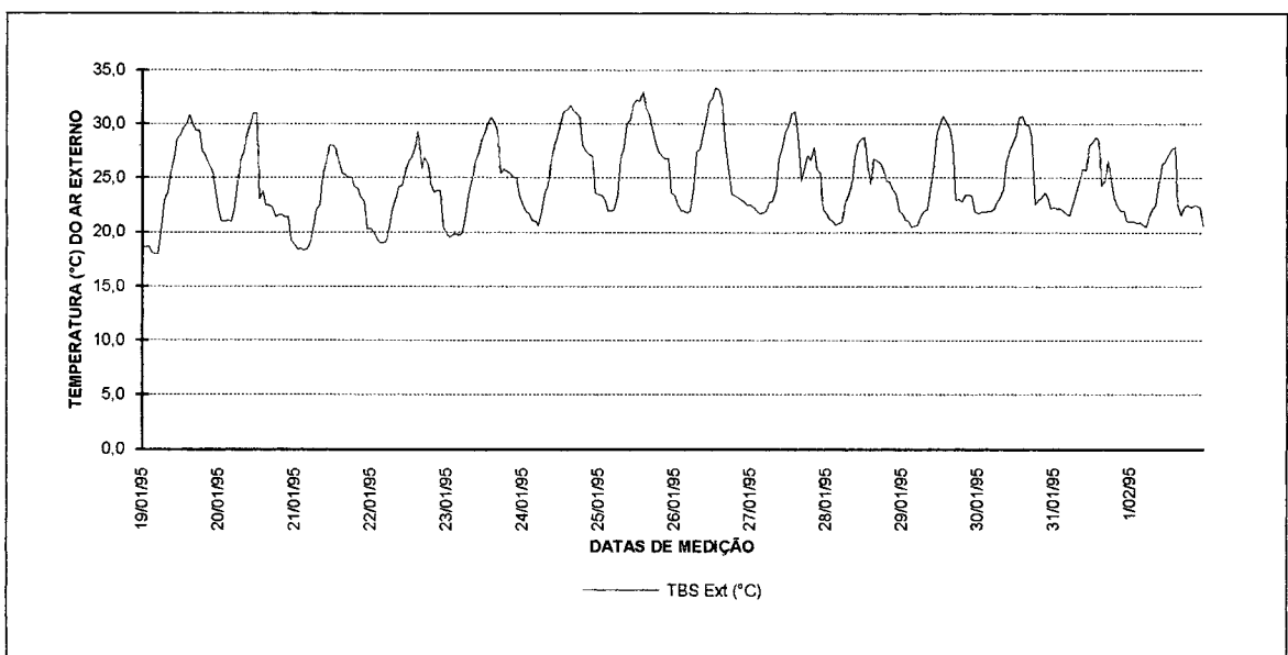
Figura 4.1 - Marcha Horária da temperatura do ar externo no verão
