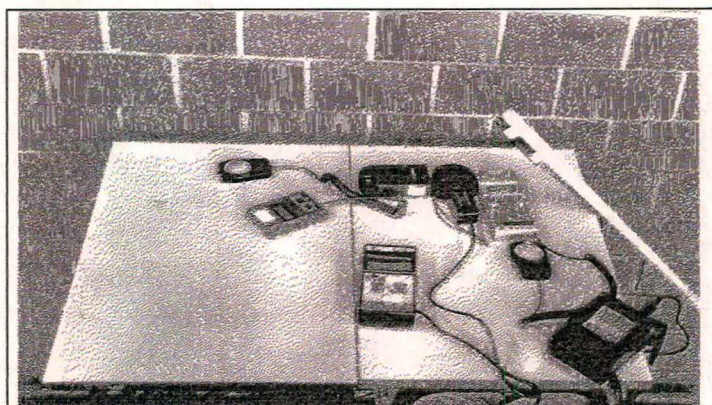
Figura 3.10 - Conjunto para a Medição Lumínica, do Vento e Temperatura Superficial
