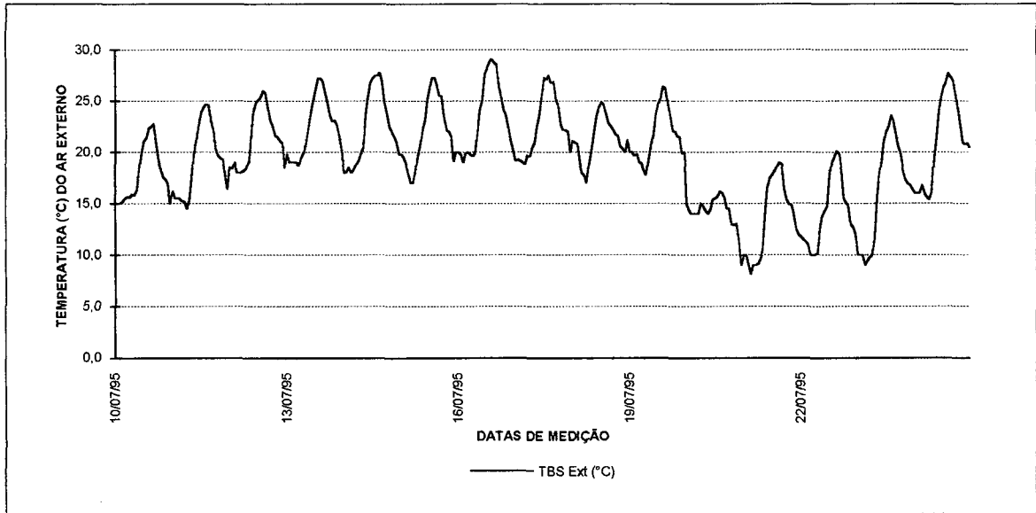
Figura 4.7 - Marcha Horária da Temperatura no Inverno.
