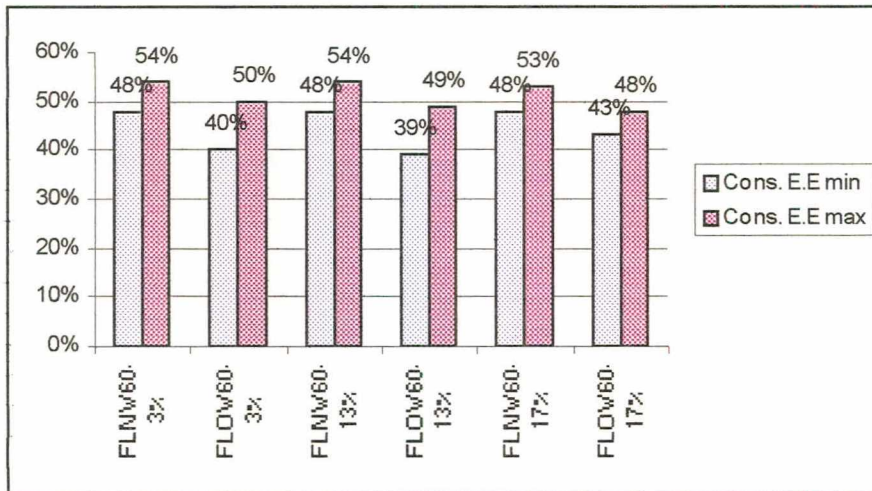
Figura 4.30 – Conservação de E E para Flamboyant (F) com luz normal (LN) e Luz Otimizada (LO) , WWR = 60% (W60), paredes externa de inércia térmica leve, orientação Norte.
