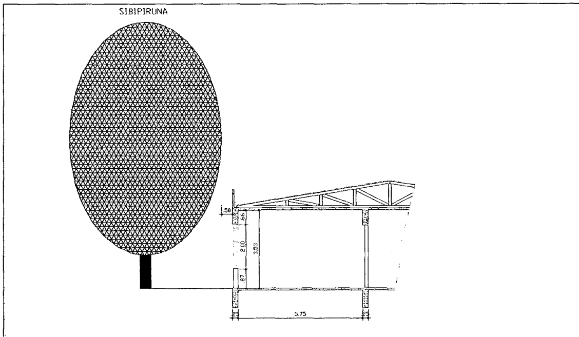
Figura 3.16 Sibipiruna adulta e o corte do Edifício
