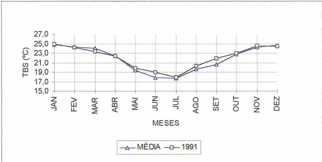
Figura 4.23 Marcha mensal das TBS (° C) da normal e do ano típico 1991
