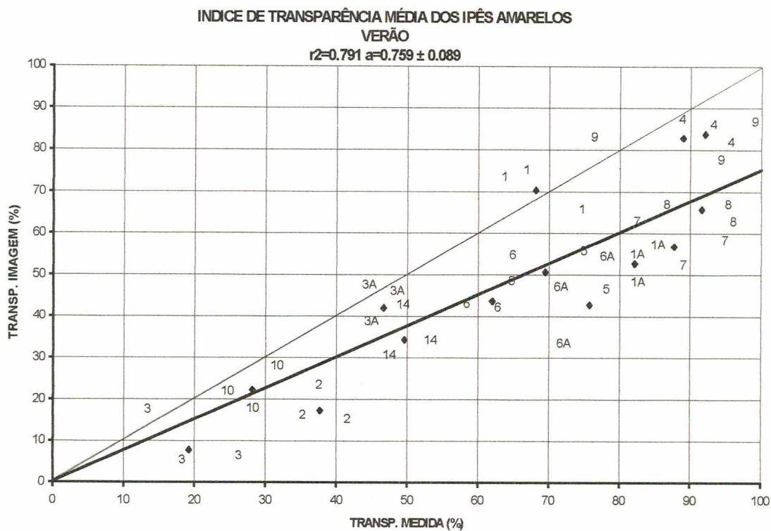
Figura 4.16 - Gráfico de correlação entre luminâncias medidas e tratamento de imagem
