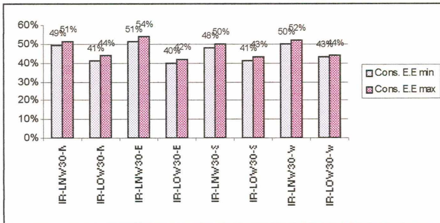
Figura 4.43 – conservação de E.E para Ipê Roxo (IR) com Luz Normal (LN) e Luz Otimizada (LO), WWR = 30% (W30), paredes externas de inércia térmica leve, todas as orientações.
