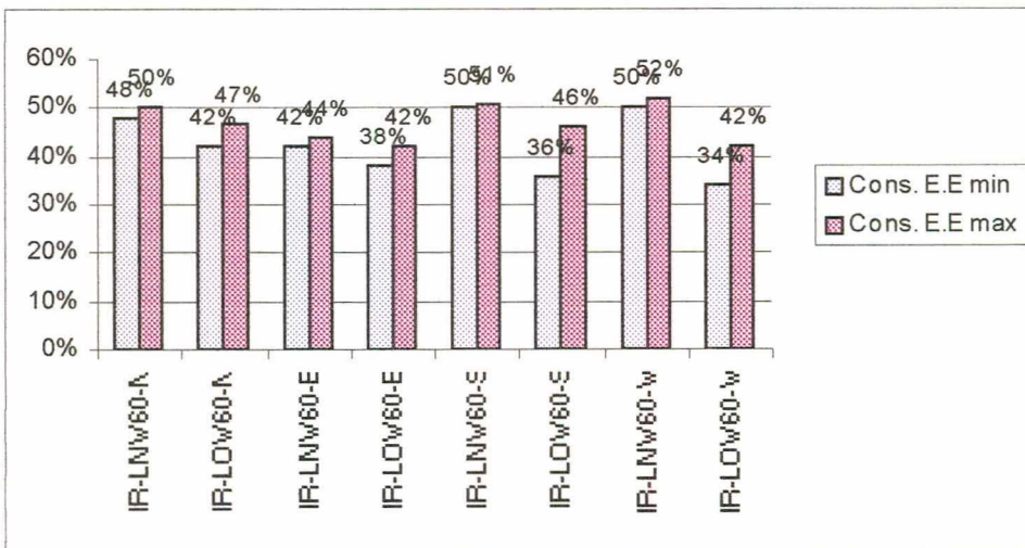
Figura 4.44 - Conservação de Ipê Roxo (IR) com Luz Normal (LN) e Luz Otimizada (LO), WWR = 60% (W60), paredes externas de inércia térmica leve, todas as orientações.
