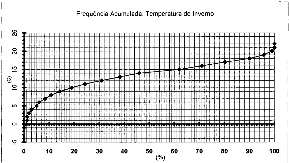
Figura 3.3. - Frequência acumulada de temperaturas mínimas para obtenção de dias típicos de Inverno, segundo PIETROBON, 1990.
