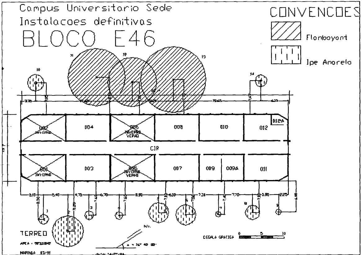
Figura 3.7. Situação Esquemática do Bloco E46 com cobertura arbórea significativa.
