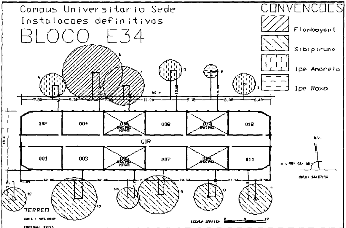
Figura 3.8. Situação Esquemática do Bloco E34 com cobertura arbórea significativa
