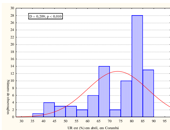
Figura 14 – Histograma da variável “ UR \text{ ext} ” em abril, em Corumbá.
