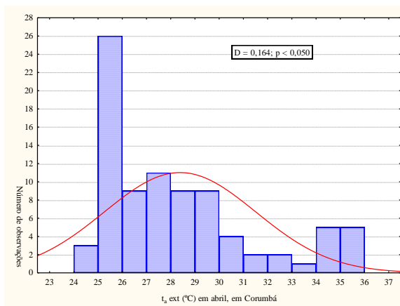
Figura 13 – Histograma da variável “ t_a \text{ ext} ” em abril, em Corumbá
