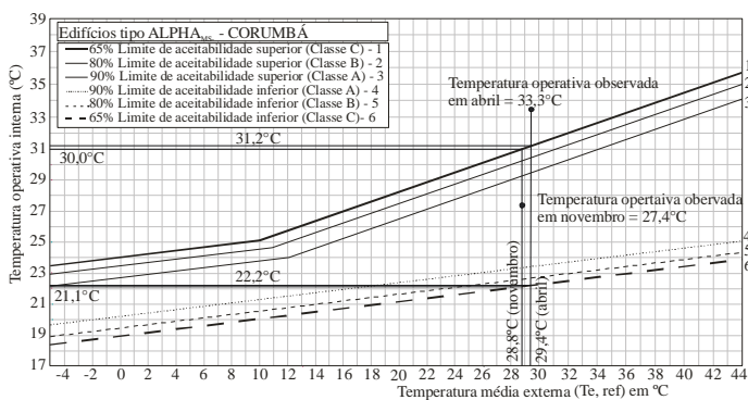
Figura 85 – Adaptive temperature limits (ATG) para ACN, em Corumbá
