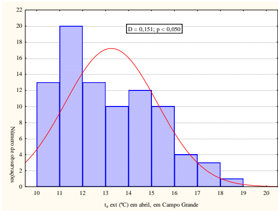
Figura 15 – Histograma da variável “t a ext” em abril, em Campo Grande.
