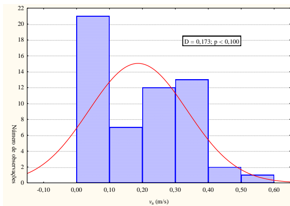
Figura 46 – Histograma da variável “v a ” em novembro, em Campo Grande
