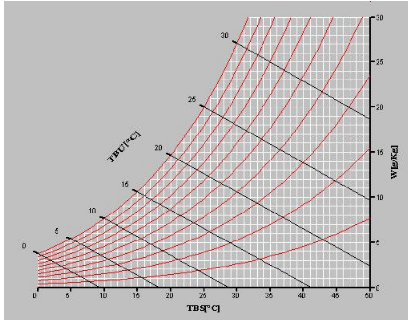
FIGURA 2.2: Modelo de carta psicrométrica
