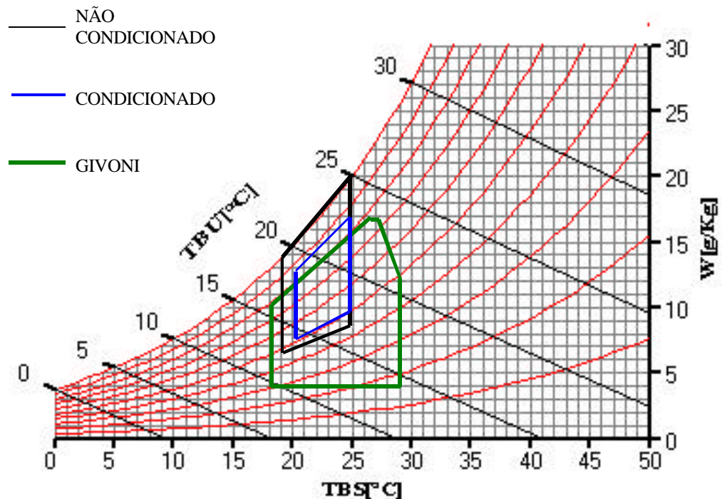
FIGURA 5.7: Desenho esquemático das zonas de conforto para ambientes em Florianópolis e a proposta de Givoni.
