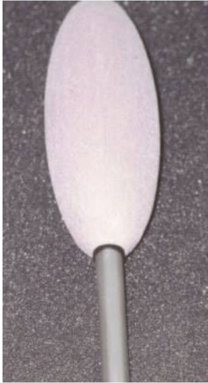
FIGURA G.9: Transdutor para medição de temperatura operativa, equipamento TYPE 1221
