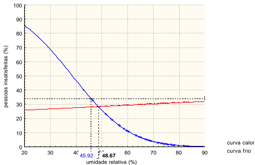
FIGURA 4.56: Curva estimadas para a umidade relativa, em prédios não condicionados, na região de Florianópolis.
