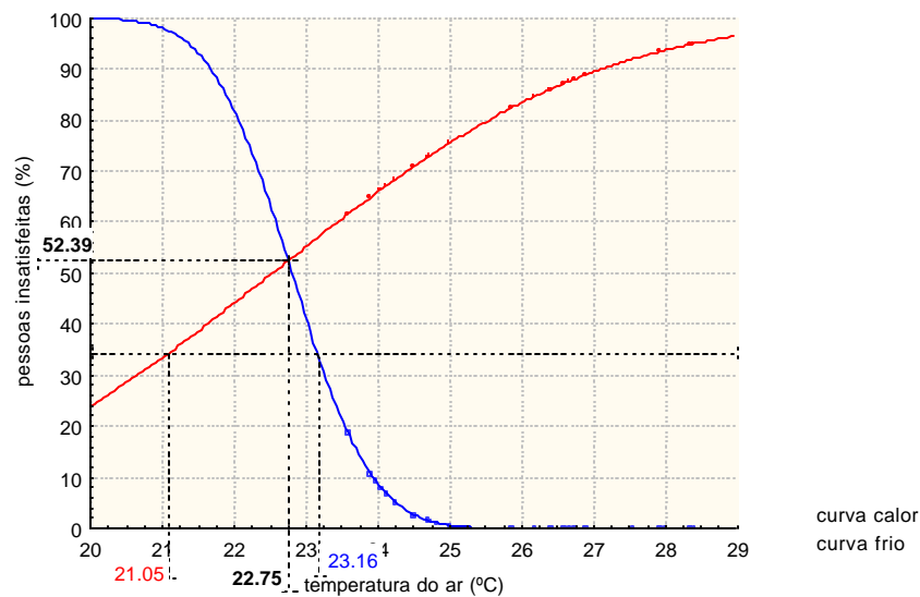
FIGURA 4.61: Curva estimadas para a temperatura do ar, em prédios condicionados, na região de Recife.
