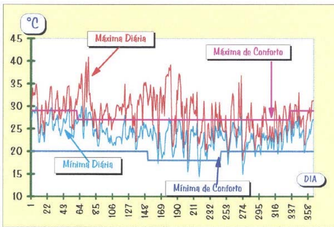
FIGURA 4.1 - Temperaturas ambientais - fachada OESTE - 25% de vidro
