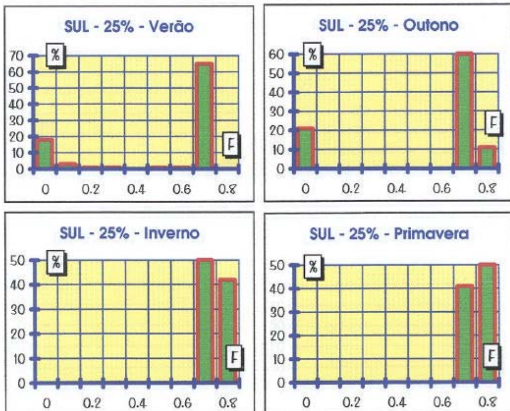
FIGURA 4.12 - Fachada SUL - 25% de janela - HISTOGRAMAS
