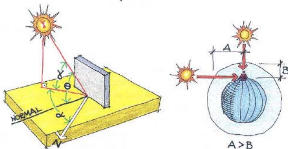
FIGURA 2.1 - Incidência da Radiação Solar
