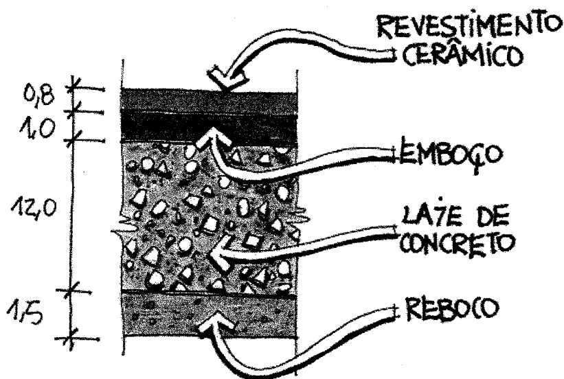
FIGURA 3.5 - Composição do piso ou teto
