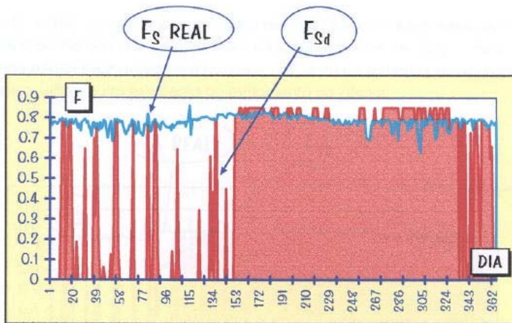
FIGURA 4.3 - Fachada NORTE - 100% de janela - F_{sd} anual
