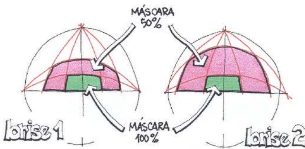
FIGURA 2.7 - Máscara de sombreamento
