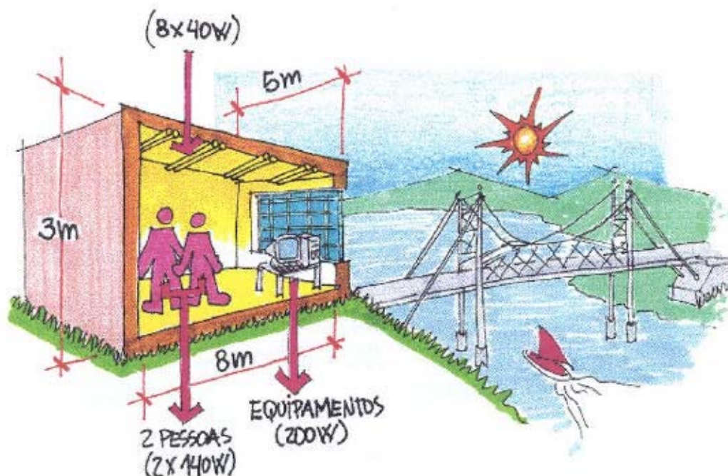
FIGURA 3.1 - Ambiente sob análise - sala comercial
