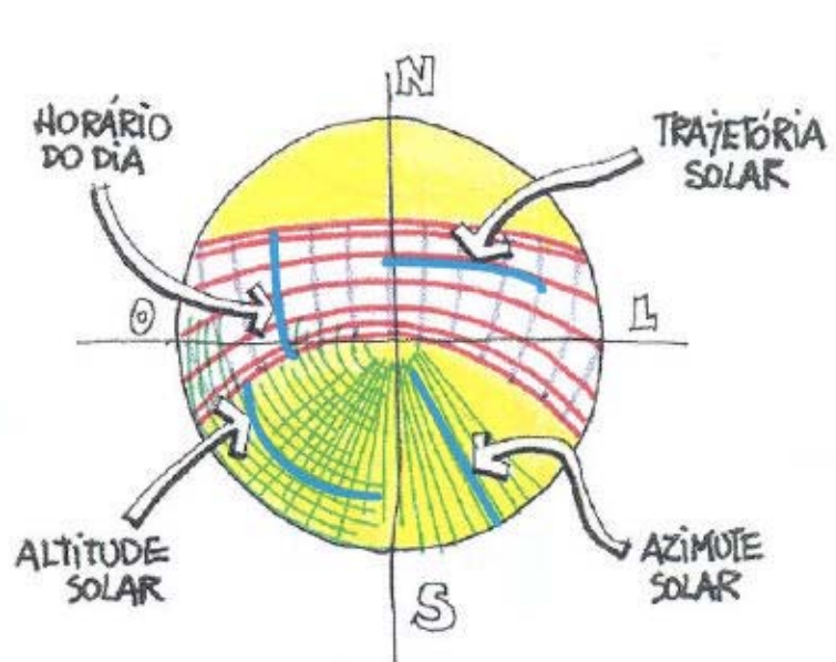
FIGURA 2.4 - Carta Solar para Florianópolis
