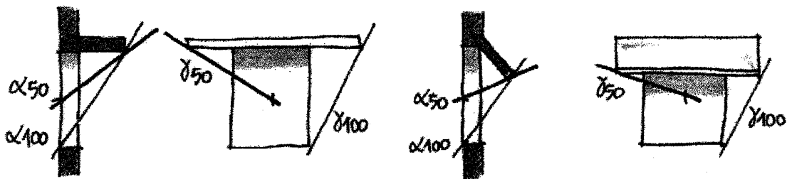
FIGURA 2.6 - Ângulos de sombreamento
