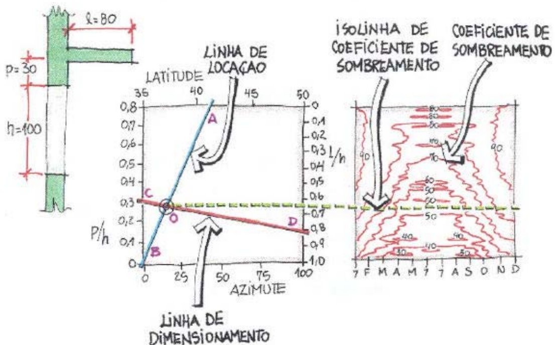
FIGURA 2.13 - Método das isolinhas
