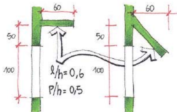
FIGURA 2.17 - Brises propostos segundo o método
