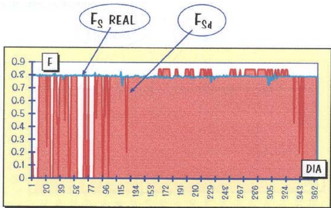
FIGURA 4.6 - Fachada LESTE - 25% de janela - F_{sd} anual
