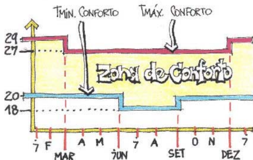
FIGURA 3.10 - Temperaturas desejáveis de conforto para os meses do ano em Florianópolis
