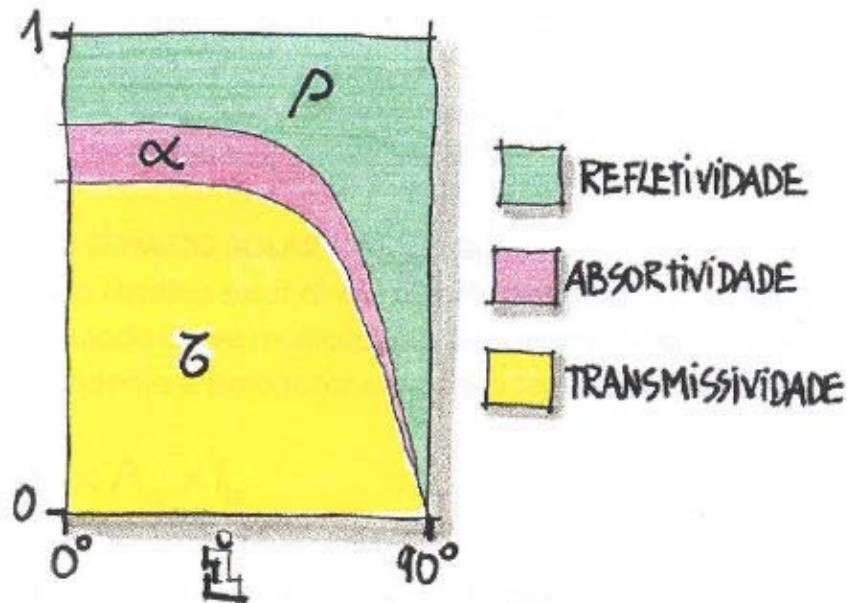
FIGURA 3.8 - Variação de \alpha , \tau e \rho com o ângulo de incidência
