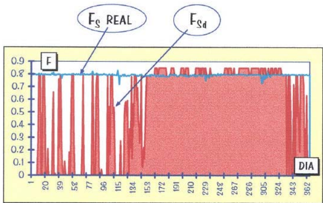
FIGURA 4.7 - Fachada LESTE - 100% de janela - F_{sd} anual
