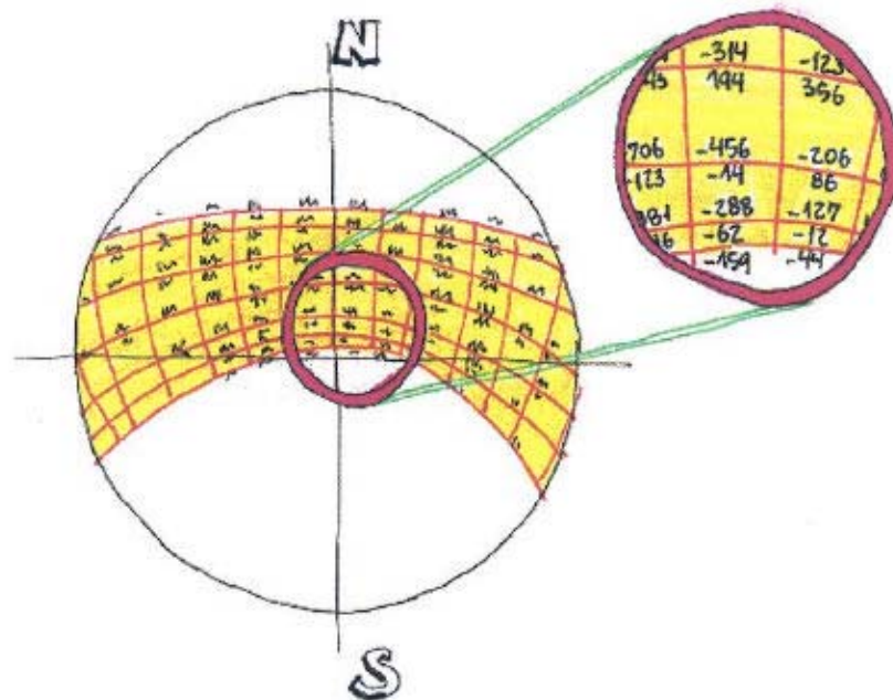
FIGURA 2.12 - Carta Solar com valores de RP para Porto Alegre
