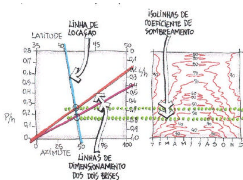
FIGURA 2.15 - Coeficientes de sombreamento dos brises estudados
