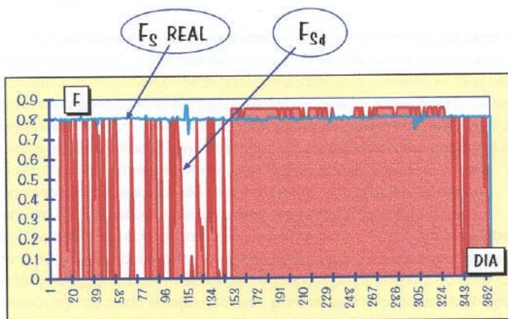
FIGURA 4.8 - Fachada OESTE - 25% de janela - F_{sd} anual
