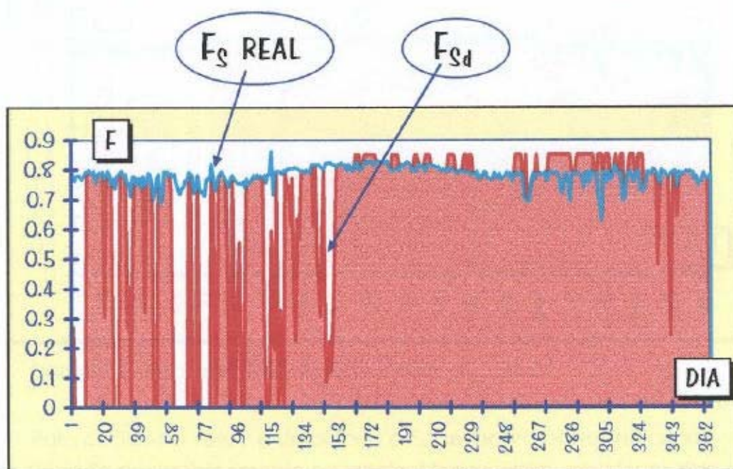
FIGURA 4.2 - Fachada NORTE - 25% de janela - F_{sd} anual
