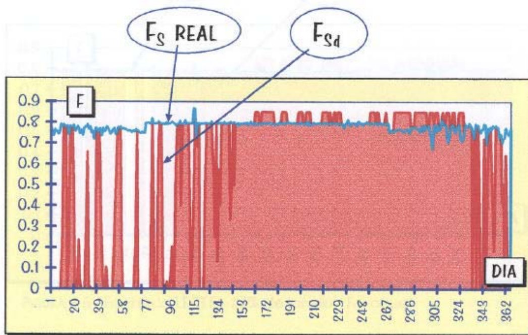
FIGURA 4.5 - Fachada SUL - 100% de janela - F_{sd} anual
