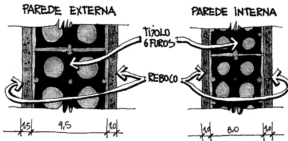
FIGURA 3.3 - Estrutura térmica média
