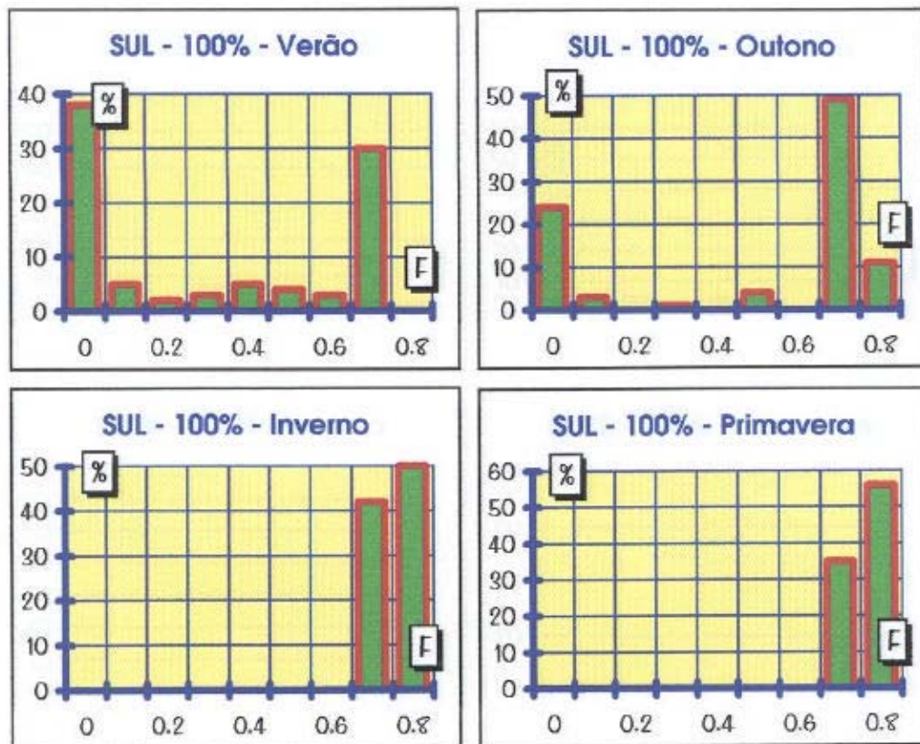
FIGURA 4.13 - Fachada SUL - 100% de janela - HISTOGRAMAS
