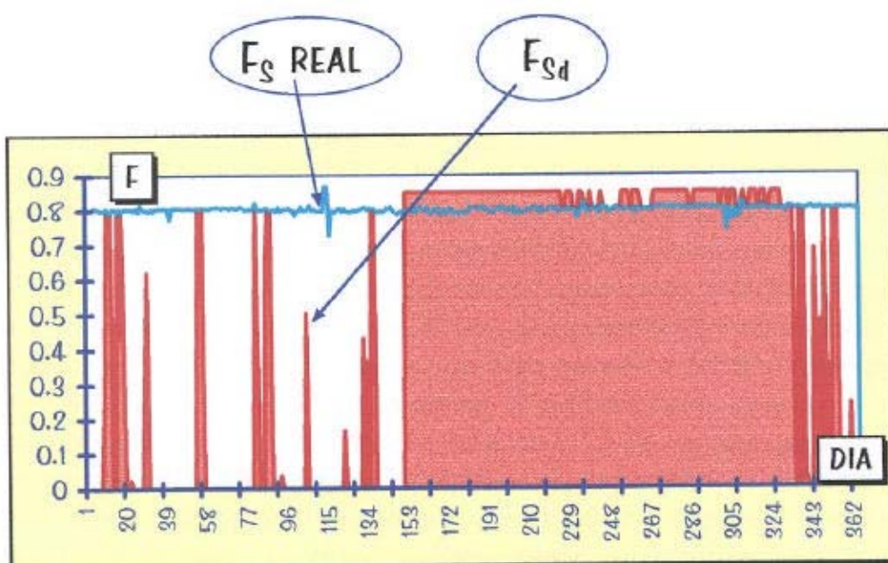
FIGURA 4.9 - Fachada OESTE - 100% de janela - F_{sd} anual
