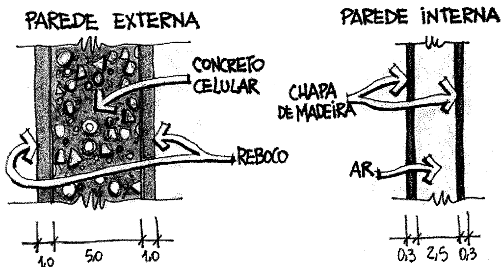
FIGURA 3.2 - Estrutura térmica leve
