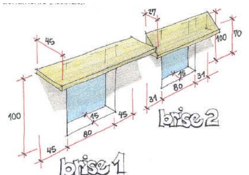
FIGURA 2.3 - Brises aplicados aos métodos
