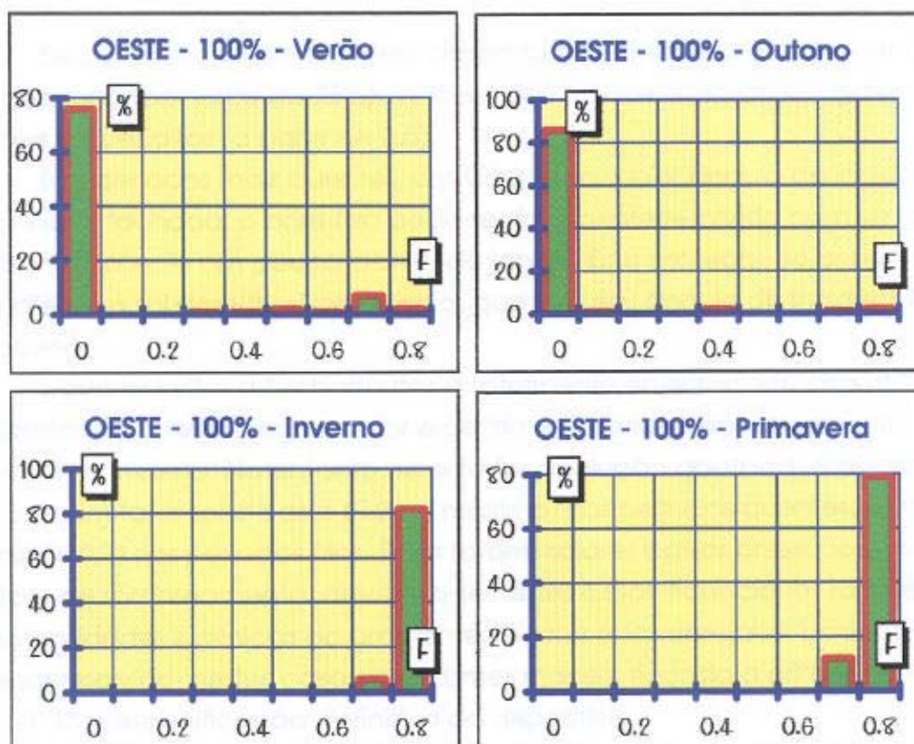
FIGURA 4.17 - Fachada OESTE - 100% de janela - HISTOGRAMAS
