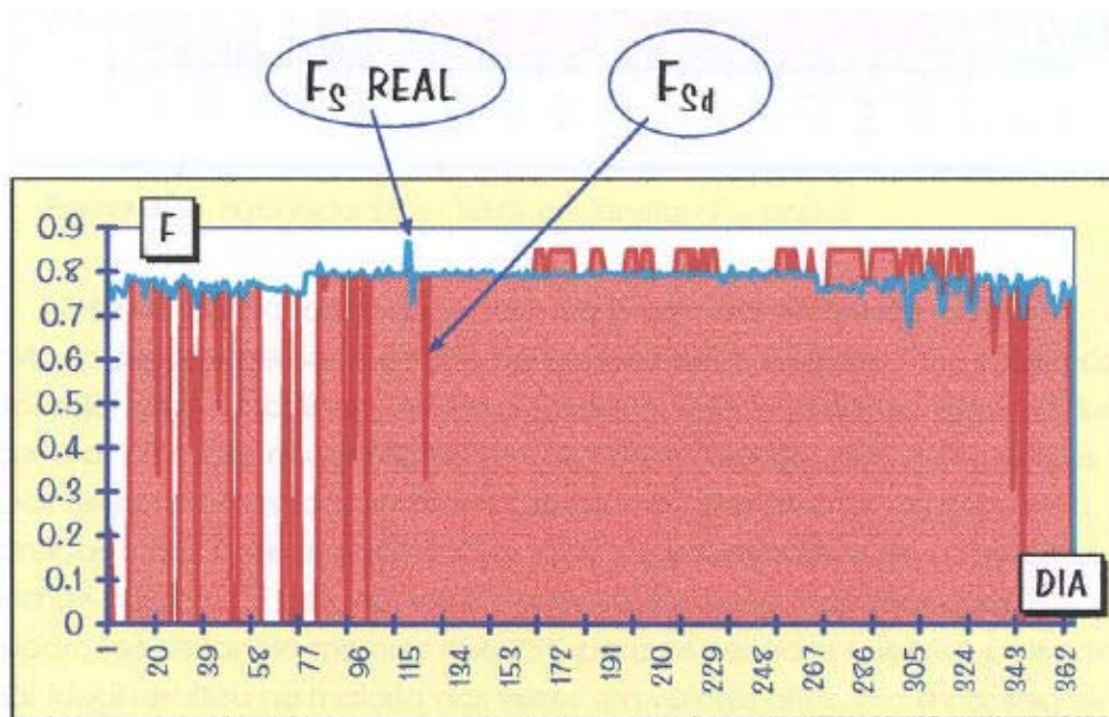
FIGURA 4.4 - Fachada SUL - 25% de janela - F_{sd} anual
