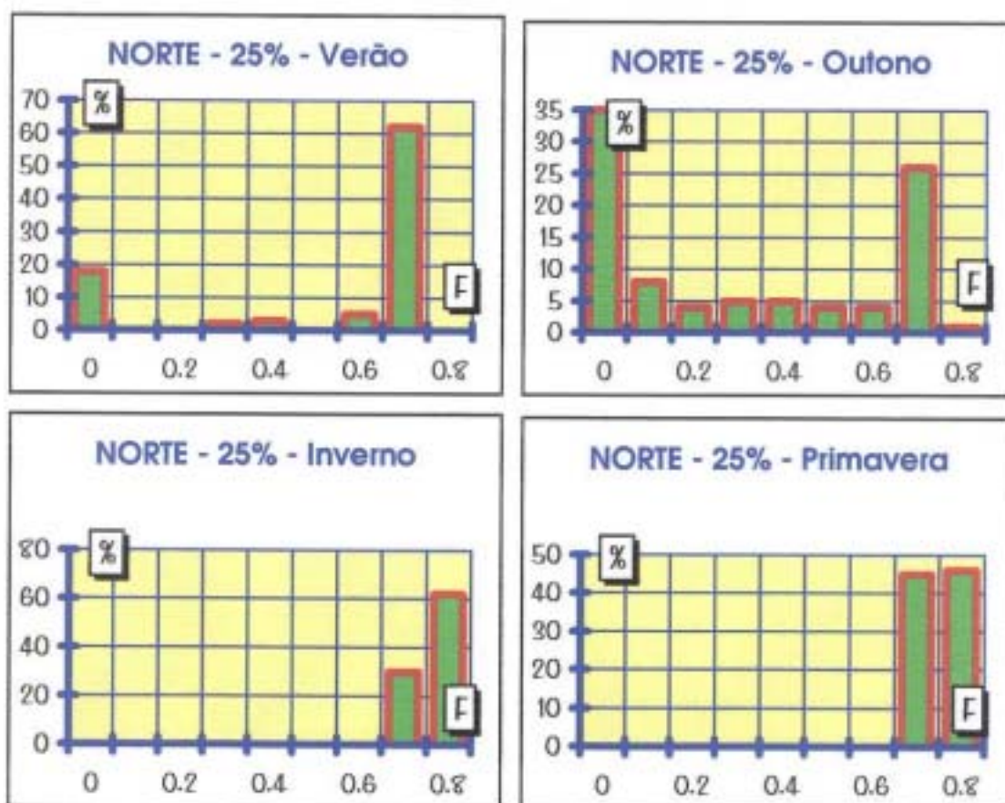
FIGURA 4.10 - Fachada NORTE - 25% de janela - HISTOGRAMAS
