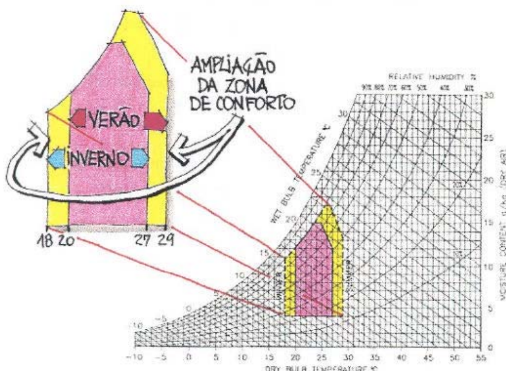
FIGURA 3.9 - Zona de Conforto de GIVONI
