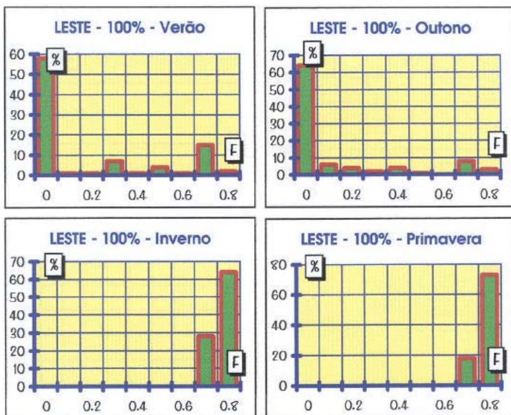
FIGURA 4.15 - Fachada LESTE - 100% de janela - HISTOGRAMAS
