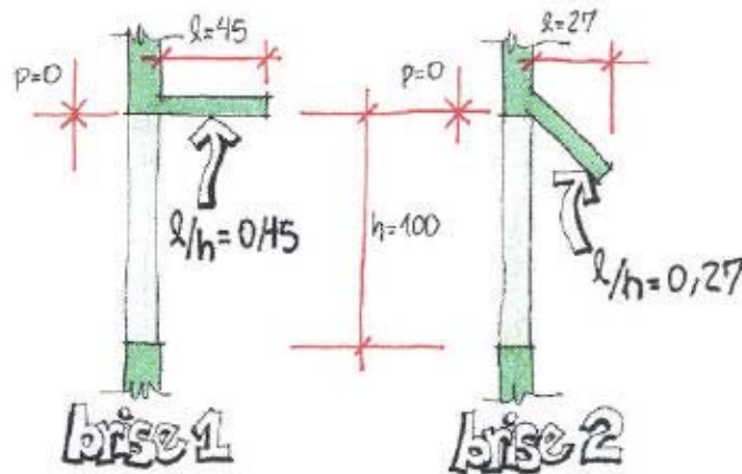
FIGURA 2.14 - Proporções l/h para os dois brises
