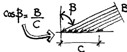
FIGURA 1.6 - Lei do cosseno
