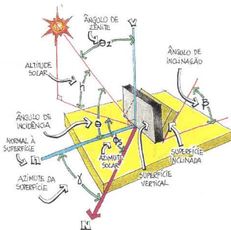
FIGURA 3.7 - Geometria solar
