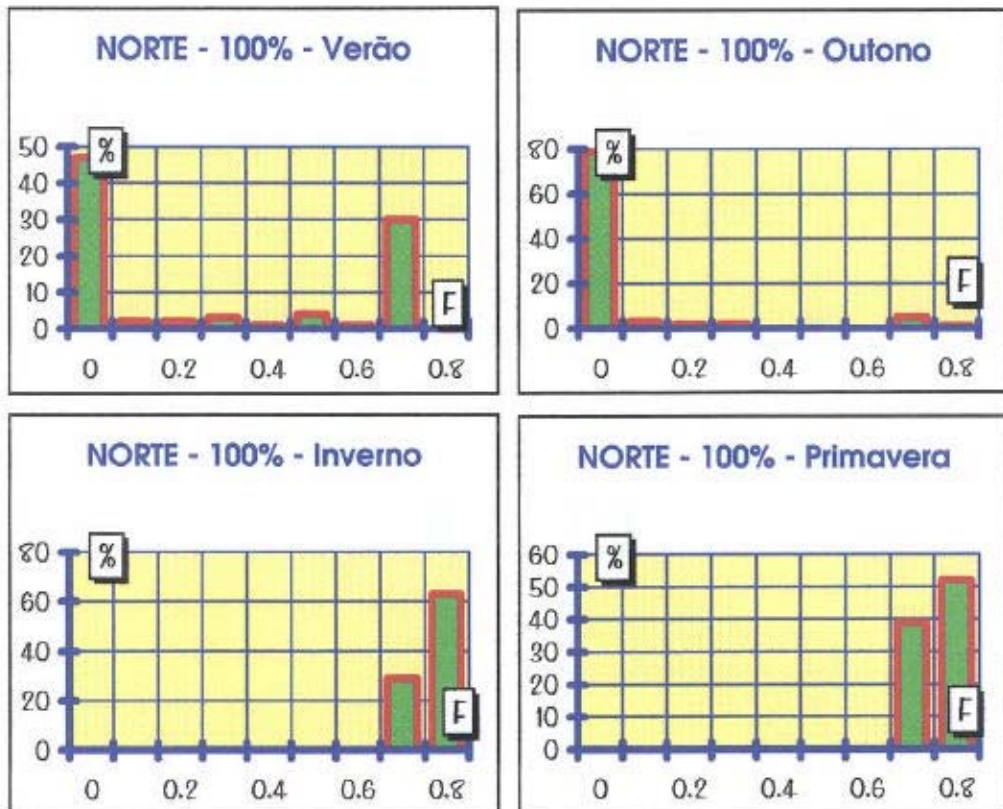
FIGURA 4.11 - Fachada NORTE - 100% de janela - HISTOGRAMAS
