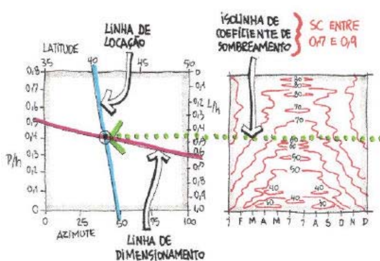
FIGURA 2.16 - Relação l/h desejável
