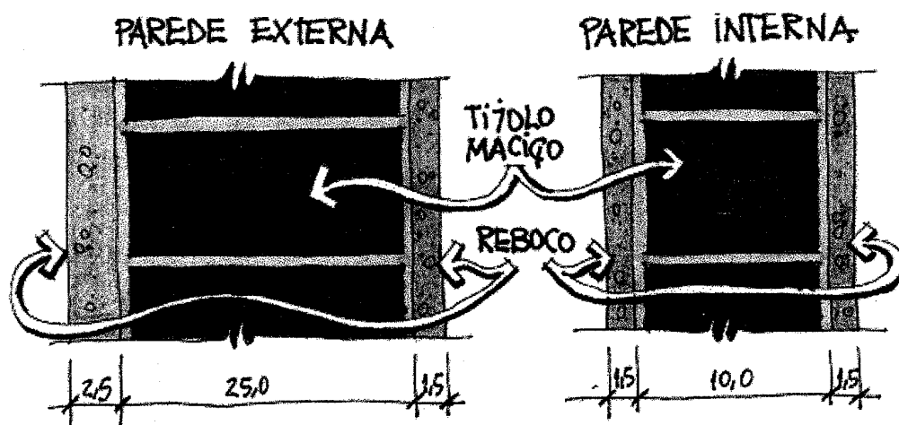
FIGURA 3.4 - Estrutura térmica pesada
