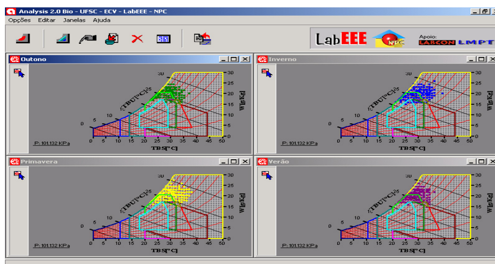
FIGURA 3.1 – Programa Analysis Bio – Carta Bioclimática para Manaus por estações do ano
