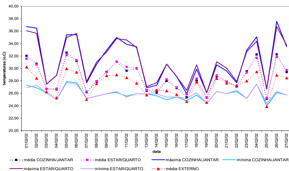
GRÁFICO 4.39 - Variações das TBS na residência 04 – 08:00/12:00 – mês de fevereiro.
