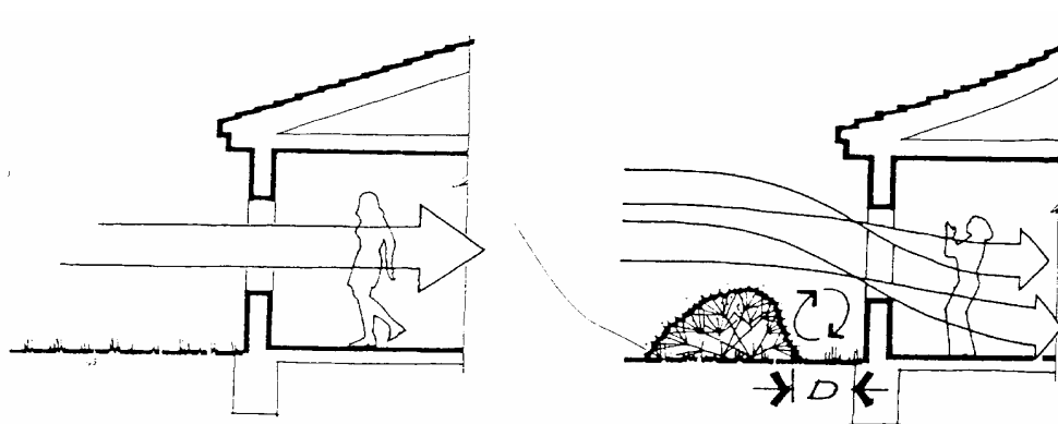
FIGURA 2.10 – Utilização de arbustos para melhorar as condições internas de conforto.
