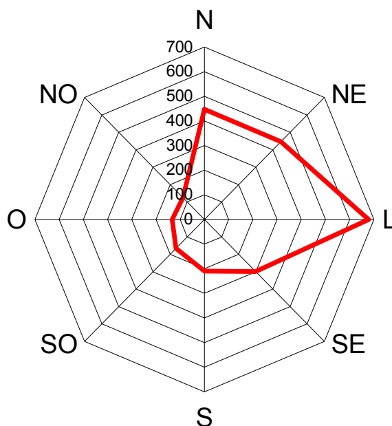
FIGURA 4.3 - Freqüência de direções dos ventos por quadrantes
