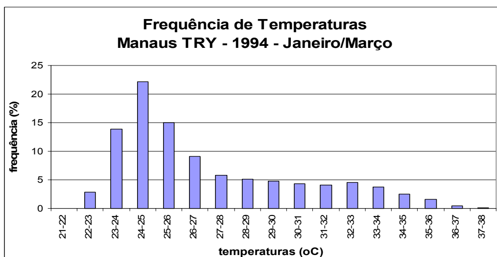
FIGURA 4.2 - Frequência de temperaturas de bulbo seco do TRY de Manaus.
