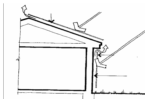
FIGURA 2.6 - Espaço entre o forro e a cobertura para eliminar a transferência de calor por convecção.
