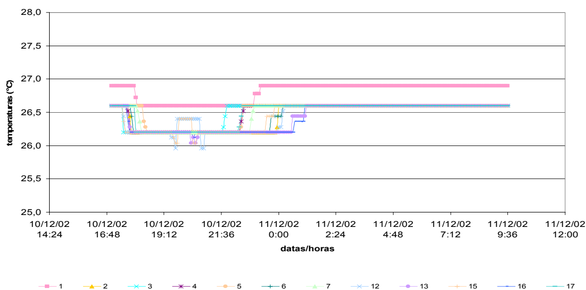
FIGURA 3.4 – Verificação da dispersão das temperaturas medidas durante a aferição dos hobsos.
