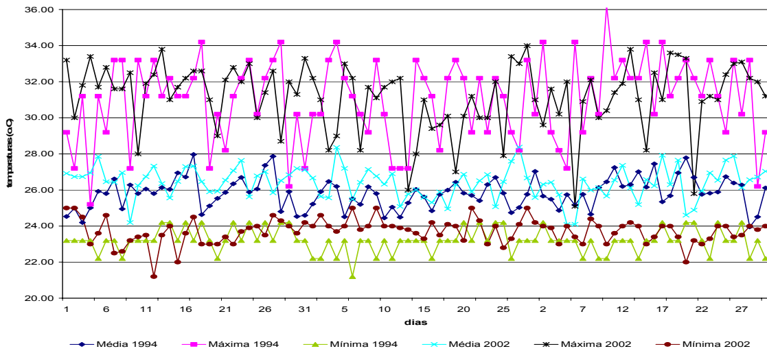
FIGURA 4.6 – Variações das TBS médias do período de janeiro à março de 1994 (TRY) e 2002..
