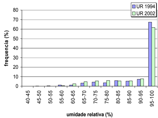
FIGURA 4.8 - Frequência de UR de janeiro a março de 2002 e do TRY de Manaus.
