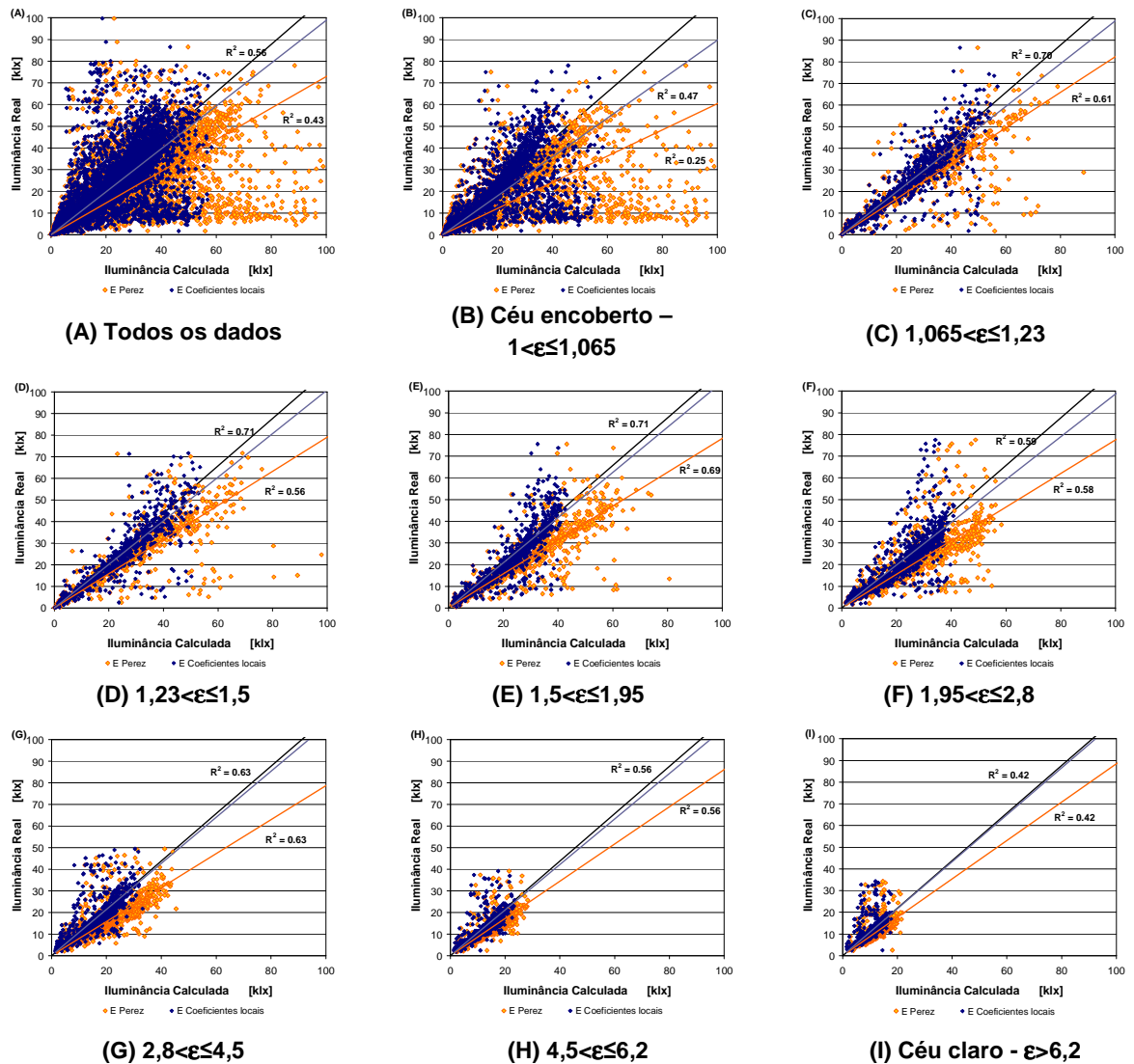
Figura 4.25. Correlação entre as iluminâncias difusas e as calculadas através dos coeficientes originais e os locais, para 2003 e 2005.
