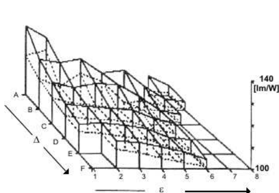
Figura 2.10. Variação da eficácia luminosa global com \Delta e \epsilon , para Z entre 35° e 50°.
