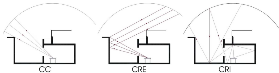
Figura 2.6. Fontes da luz natural distribuída no ambiente interno.
