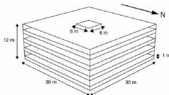
Figura 2.1. Modelo de edifício estudado, com aberturas nas quatro fachadas e lanternim, e refletâncias iguais a: paredes - 0,5; piso - 0,3; e teto - 0,7.
