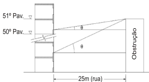
Figura 2.27. Definição do ângulo de obstrução externa
