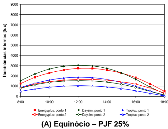
Figura 4.6. Valores das iluminâncias internas para o modelo com PPF de 25%, proporção 1:1, refletância das paredes e teto de 0,85 e piso de 0,60; para Florianópolis.
