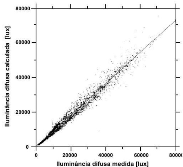
Figura 2.19. Correlação entre iluminâncias difusas modeladas e medidas de Nova Zelândia.
