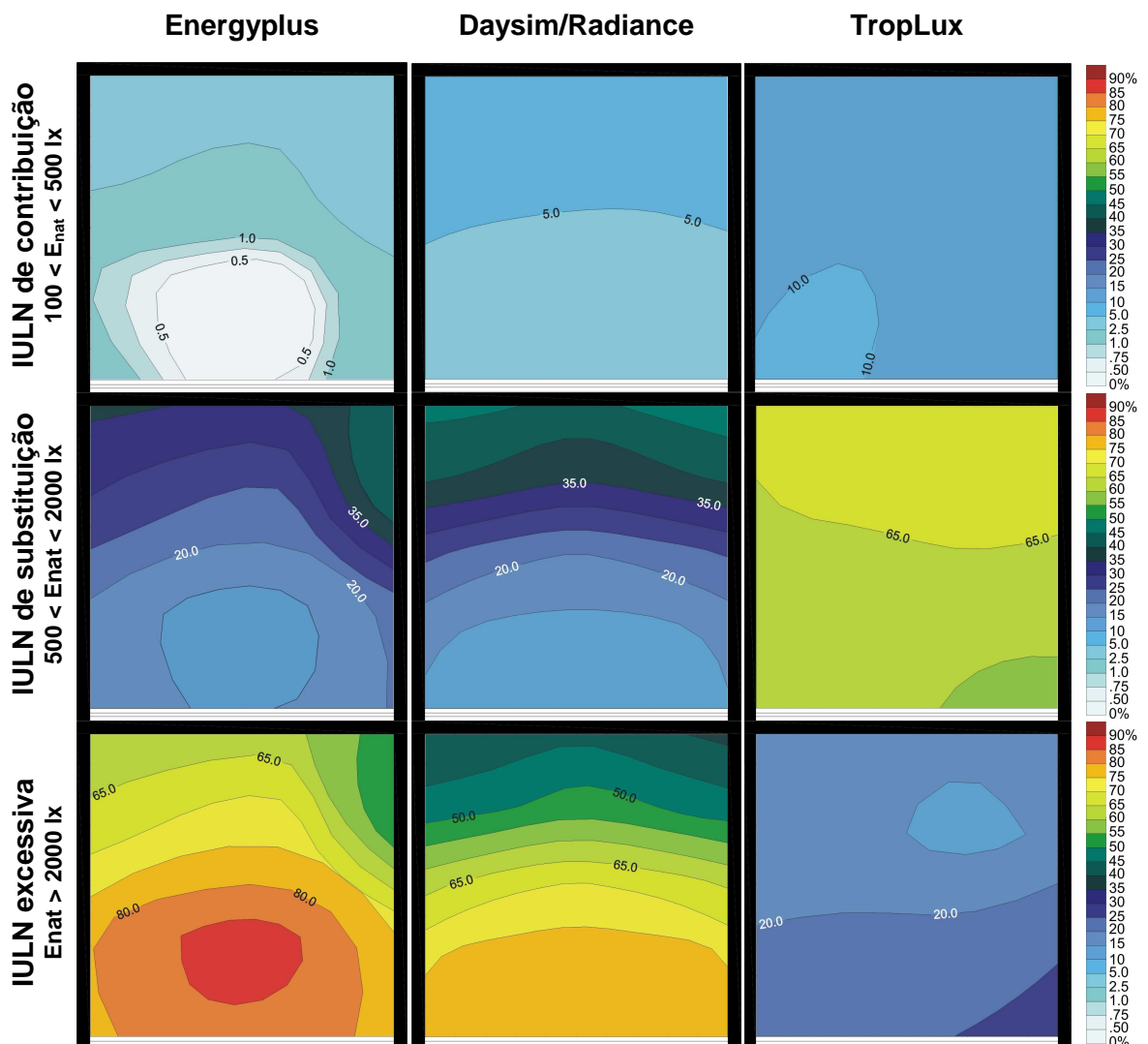
Figura 4.1. IULN calculada através da simulação da iluminação natural, para sala com: PJJ de 50%, refletância das paredes e teto de 0,85 e piso de 0,60; para Florianópolis.
