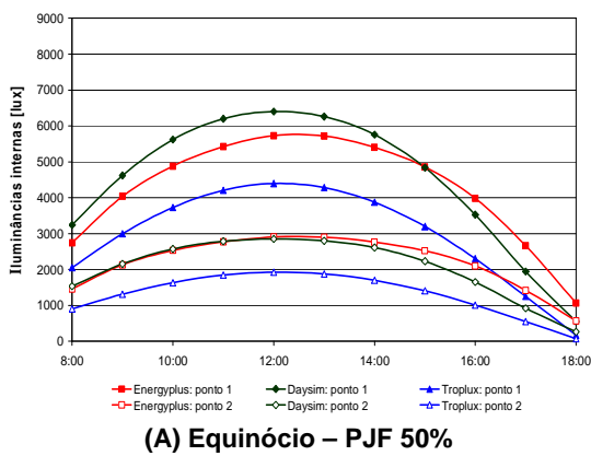
Figura 4.7. Valores das iluminâncias internas para o modelo com PPF de 50%, proporção 1:1, refletância das paredes e teto de 0,85 e piso de 0,60; para Florianópolis.
