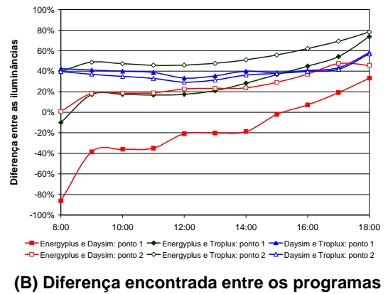
Figura 4.6. Valores das iluminâncias internas para o modelo com PPF de 25%, proporção 1:1, refletância das paredes e teto de 0,85 e piso de 0,60; para Florianópolis.
