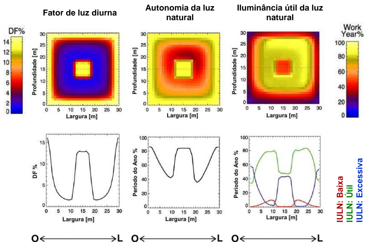
Figura 2.2. Gráficos de Fator de Luz Diurna, Autonomia da luz natural e Iluminância Útil da Luz Natural.
