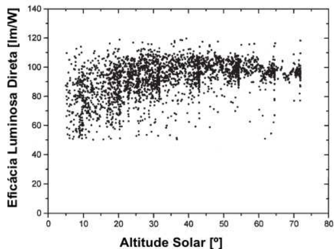
Figura 2.7. Eficácia luminosa direta em função da altura solar para todos os tipos de céu.
