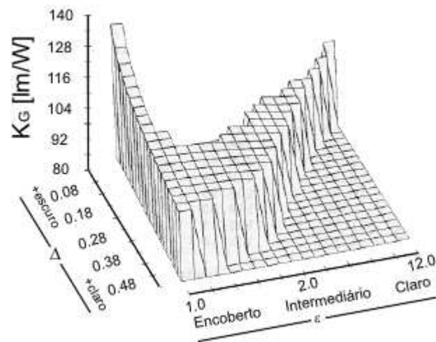
Figura 2.13. Superfície Polinomial com variação da eficácia luminosa global ( K_G ) em função da claridade do céu ( \epsilon ) e brilho do céu ( \Delta ), para ângulo zenital e temperatura constantes.
