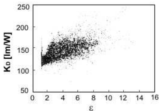
Figura 2.14. Variação da eficácia luminosa difusa ( K_D ) em função da claridade do céu.
