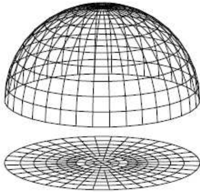
Figura 2.4. Hemisféra de raio unitário.
