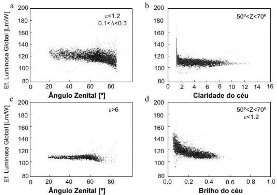
Figura 2.12. Variações da eficácia global em função de: a. ângulo zenital para condições céu encoberto; b. claridade do céu para um ângulo zenital limitado; c. ângulo zenital para céu claro e, d. brilho do céu para céu encoberto. Com dados de Nova Iorque e Genebra.
