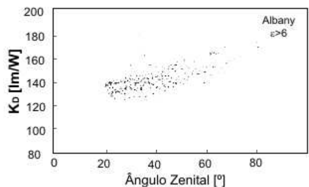
Figura 2.15. Variação da eficácia luminosa difusa ( K_D ) para dados de Albany, em função do ângulo zenital para céu claro.
