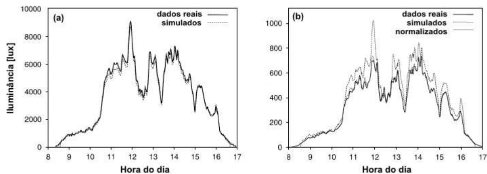
Figura 2.31. Iluminâncias externa (a) e internas com a veneziana aberta (b), para condição de céu encoberto.
