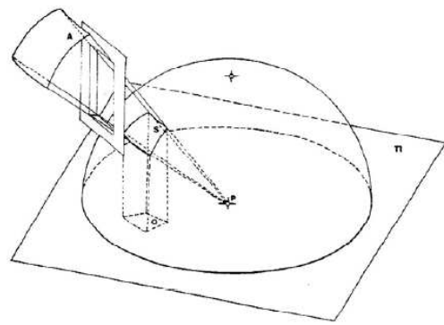
Figura 2.4. Hemisféra de raio unitário.
